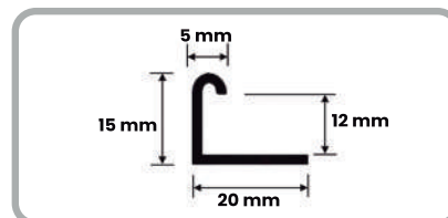
Comprimento: 120 cm Composição: Aço Inox 304
